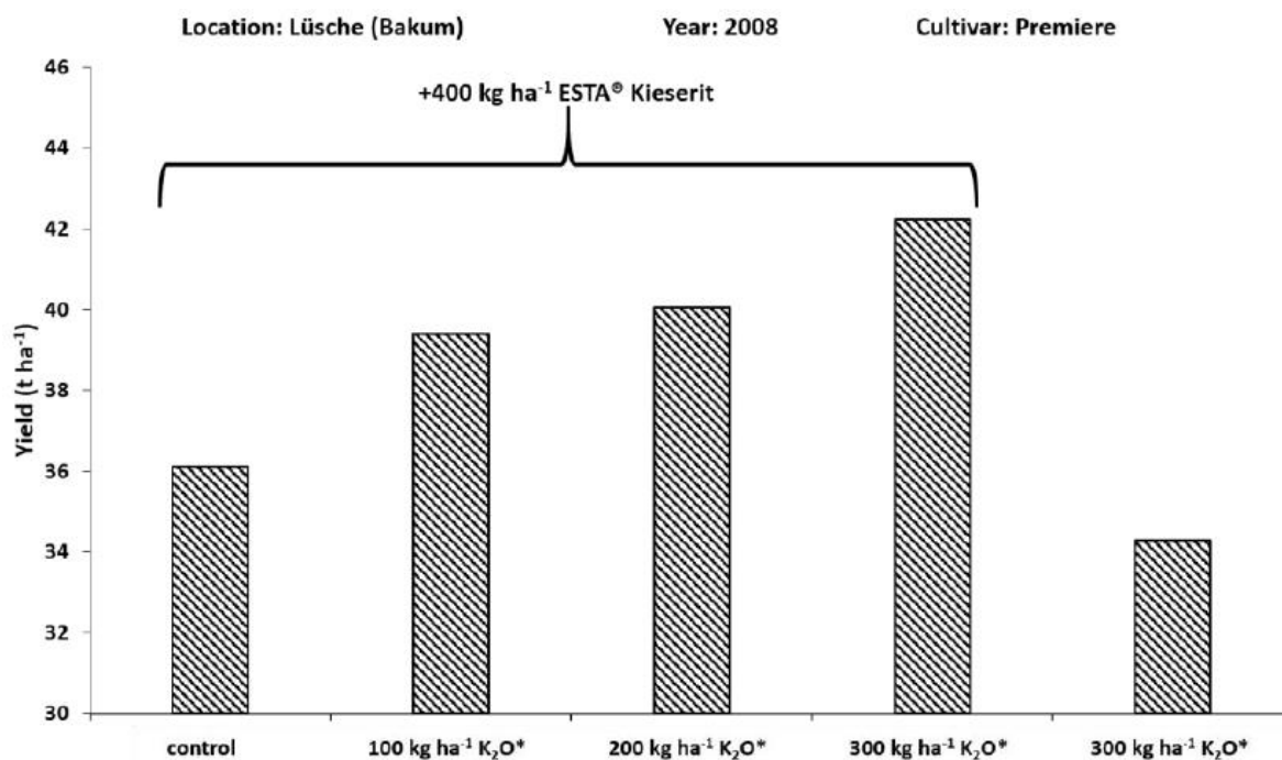
Figuur 6 Het effect van een gecombineerde K- en Mg-bemesting op de opbrengst van aardappel in Noordwest-Duitsland op slibachtig zand met 13,6 mg K 2 O 100 g -1 (CAL- extractie) en 3,2 mg Mg/100 g -1 (CaCl 2 -extractie) in de bodem. Magnesium werd toegediend als; ESTA® Kieserit en kalium als kaliumsulfaat (KALISOP®). De bodemwaarden worden herleid naar Handboek bodem en bemesting als laag gekwalificeerd.
