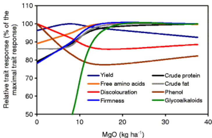
Figuur 4. Opbrengst- en kwaliteitsparameters die worden beïnvloed door de levering van Mg aan aardappel (schematisch). Voor elke parameter die in de grafiek is weergegeven, zijn de waarden berekend ten opzichte van hun maximale expressie (= 100 %) aan Mg-levering. Bron: Gerendás & Führs (2011) en gebaseerd op: Evans en Mondy 1984; Klein et al. 1981 & 1982).
